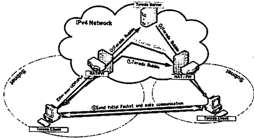
図 6: Teredo クライアント間の通信
