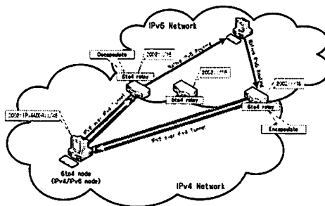
図 2: 6to4 ノードと IPv6 ホストの通信
