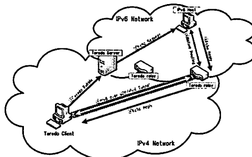
図 5: Teredo クライアントから IPv6 ホストへの通信
