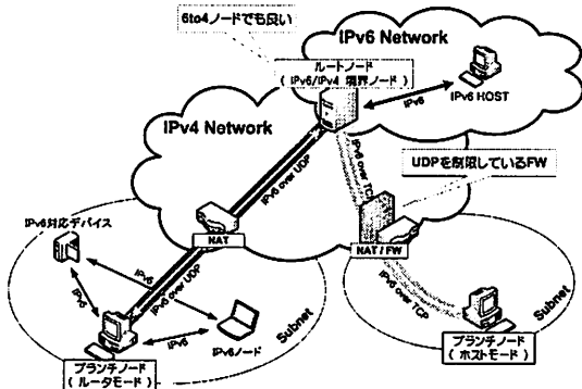
図7: ルートノードとブランチノード
