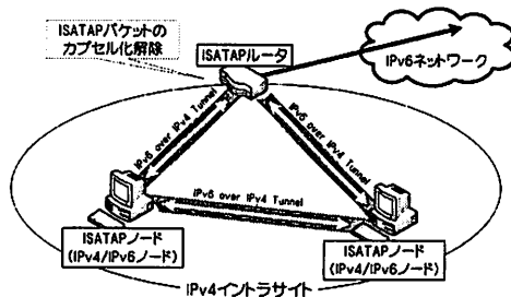
図 3: ISATAP のルーティング
