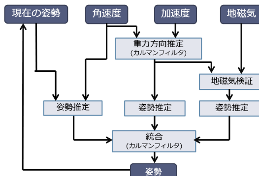
図2: 姿勢推定のフローチャート
