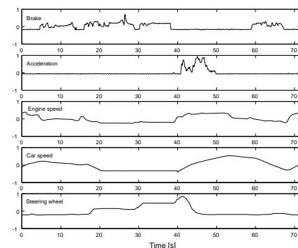
図 2: 運転行動データの記録例: 上からブレーキ踏力、アクセル踏力、エンジン回転数、車速、ハンドル切り角
